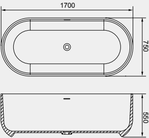
B0301 Bathtub 浴缸 尺寸：1700×750×550mm
