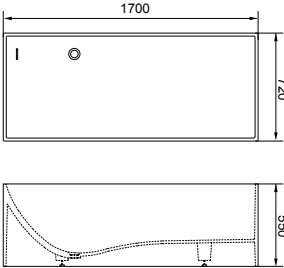
B0306 Bathtub 浴缸 尺寸：1700×720×550mm
